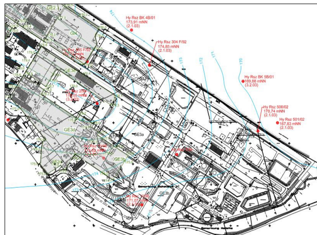
Auszug aus Isohypsenplan des oberen GW-Leiters
