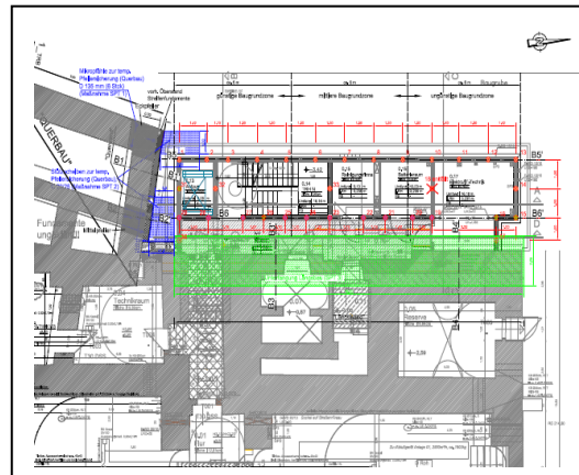
Lageplan der Spezialtiefbaumaßnahmen
