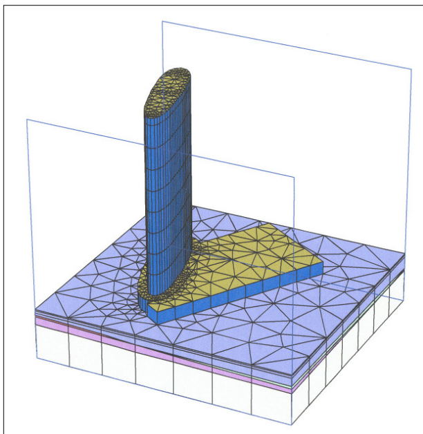
FEM-Modell des JUSAO-Towers
