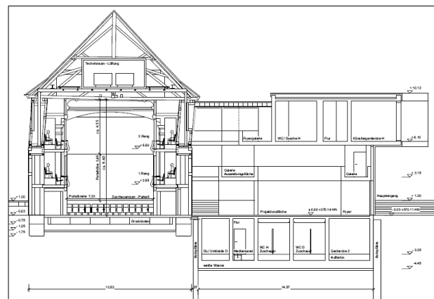
Querschnitt Kerngebäude und Erweiterungsbau
