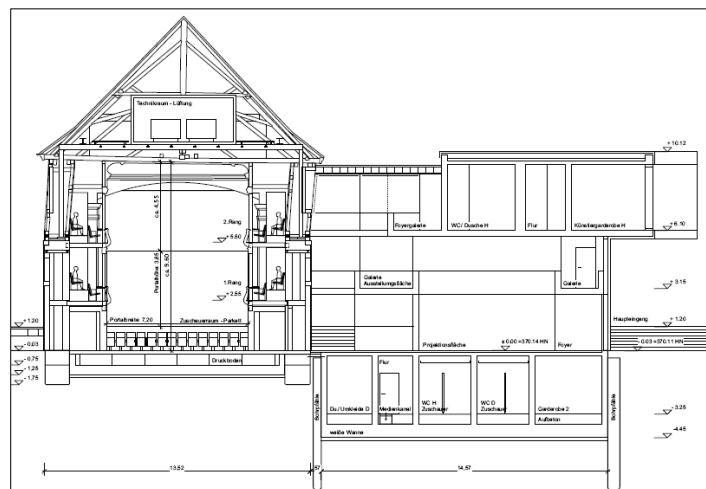
Querschnitt Kerngebäude und Erweiterungsbau
