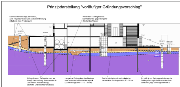
Prinzipdarstellung „vorläufiger Gründungsvorschlag“
