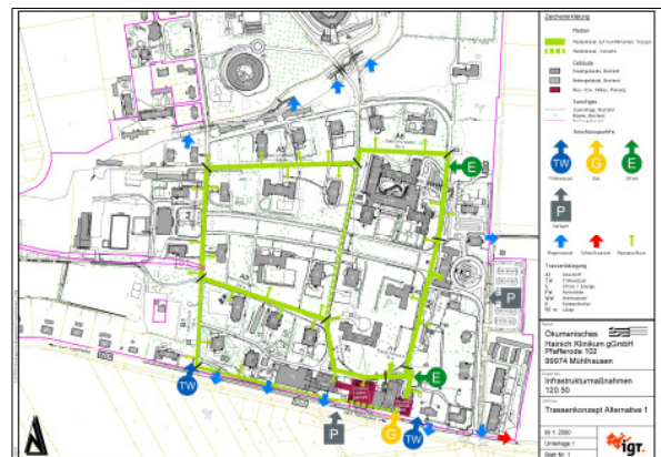
Übersichtsplan Innere Erschließung
